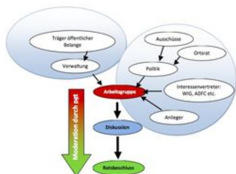
Ablaufplan Leitbildprozess
